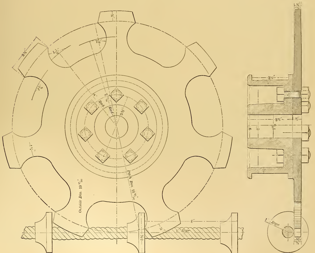
FIG. 4.—SPROCKET WHEEL.
